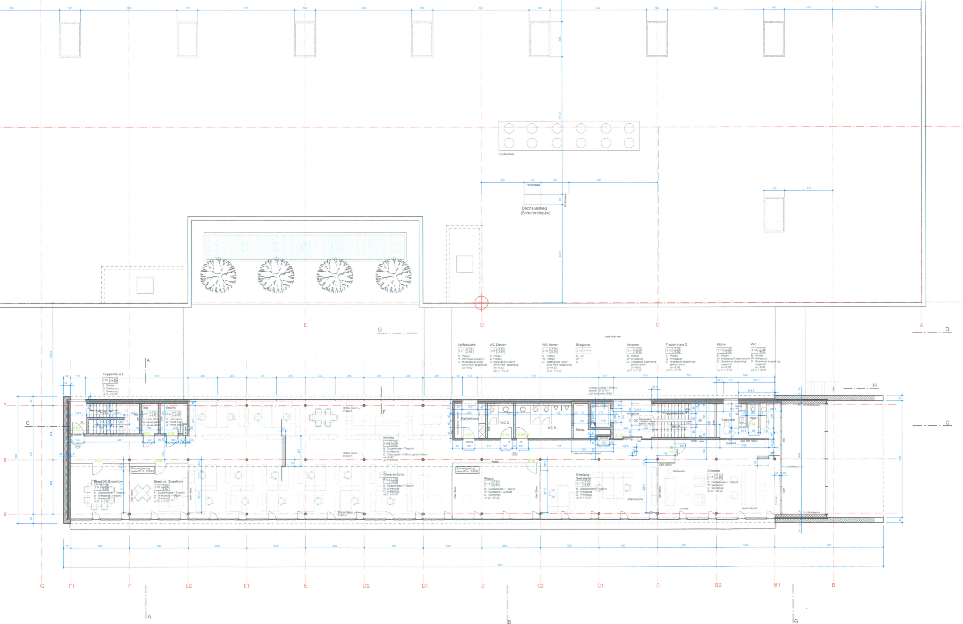
2. Obergeschoss
